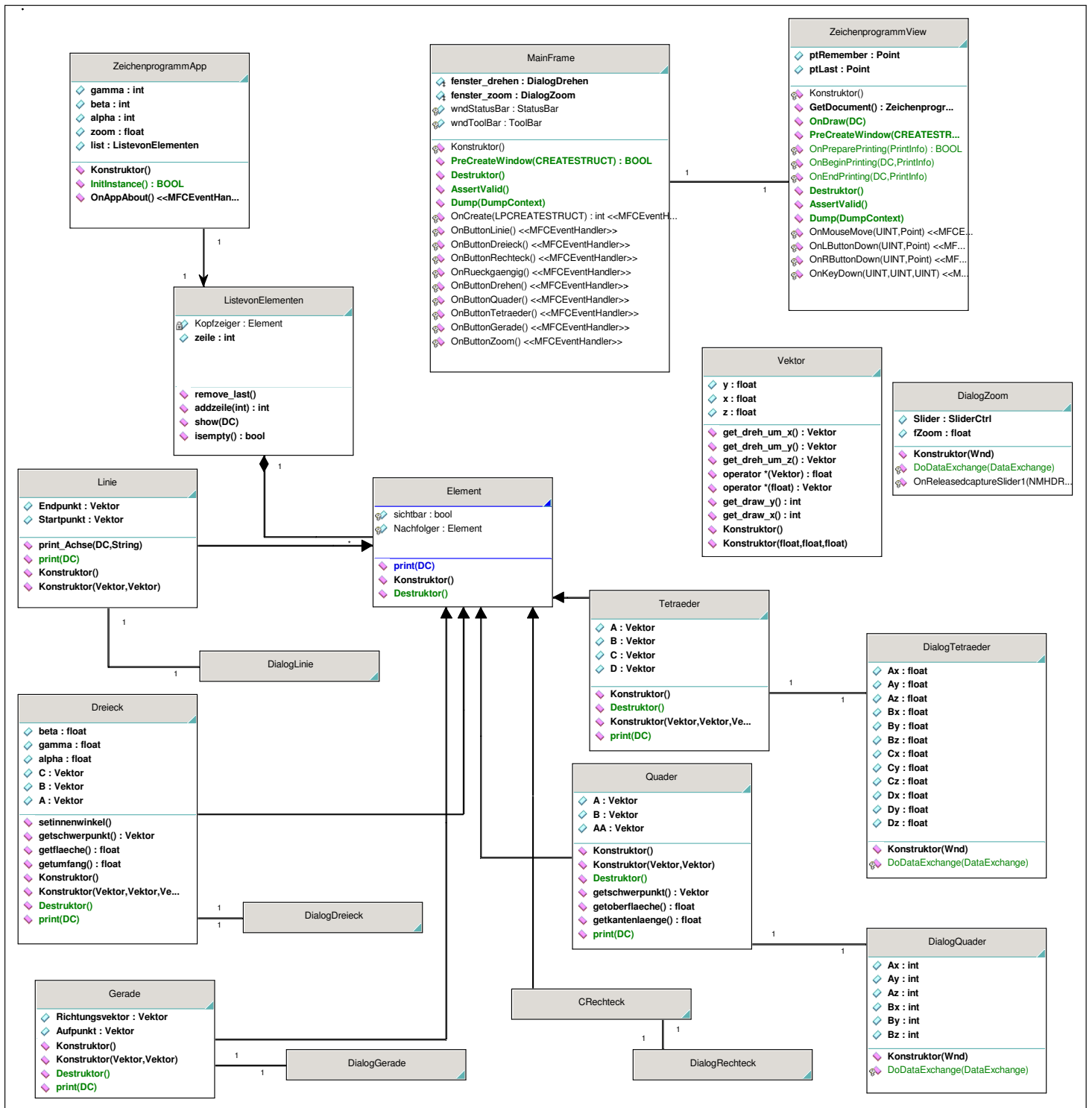
Zeichenprogramm
